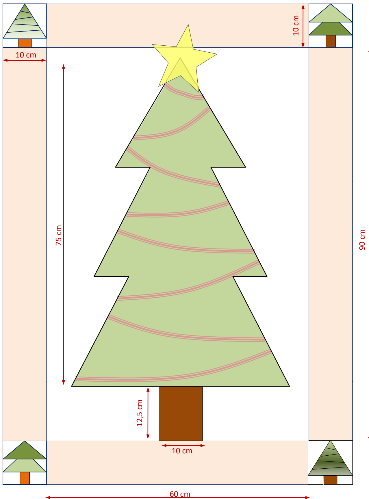
Esquema del Calendario (sin adornos colgantes) (Dibujo hecho a escala 1:5)
